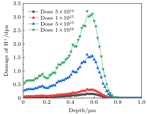
图 3 不同剂量 \text{H}^+ 离子辐照离位损伤
