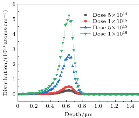
图 2 \text{H}^+ 离子辐照深度
