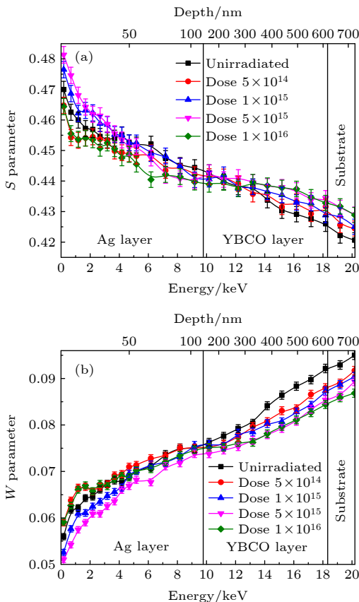
图 4 不同剂量 H^+ 离子辐照前后, 样品 S 参数及 W 参数随正电子入射能量的变化关系
