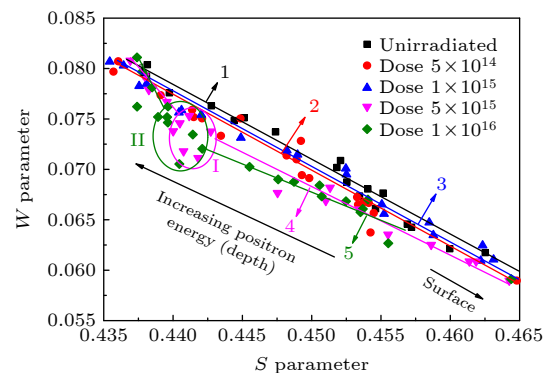
图 5 不同剂量 H^+ 离子辐照前后样品的 S 参数随 W 参数的变化关系
