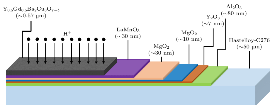
图 1 超导带材结构
