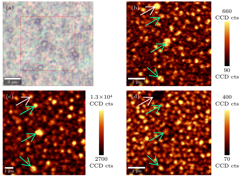
图 5 样品 S3 的面扫描结果 (a) 样品面扫描测试区域为红框所示 10\ \mu\text{m}\times 10\ \mu\text{m} 区域, 测试步长为 100\ \text{nm} ; (b) 以 1332\ \text{cm}^{-1} (金刚石) 为中心的拉曼面扫描结果; (c) 以 738\ \text{nm} (金刚石硅空位色心) 为中心的 PL 面扫描结果; (d) 以 520.7\ \text{cm}^{-1} (硅单质) 为中心的拉曼面扫描结果; 箭头指出了几个晶粒在各图当中的位置, 从光谱看白色箭头所指的晶粒无硅单质信号, 绿色箭头所指的晶粒既有硅单质信号也有硅空位色心信号
