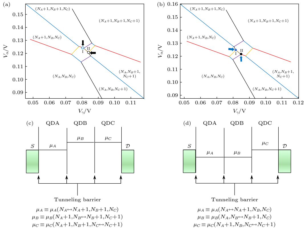
图 5 第二类三点, 其中 I 区指代的是 (N_A, N_B+1, N_C) 区域, II 区指代的是 (N_A+1, N_B, N_C+1) 区域 (a) 对应了图 3 中的蓝色虚线方框, 这里 V_\beta = 0.0106 V. 箭头指代的空心点标示了在该三点处是空穴型输运; (b) V_\beta = 0.0078 V. 箭头指代的实心点标示了在该三点处是电子型输运. 图 (b) 对应二维稳态图的 V_\beta 值小于图 (a) 的 V_\beta 值; (c) 图 (a) 蓝色空心点对应的电化学势对齐情况, QDA, QDB 和 QDC 分别指代的是量子点 A, B 和 C; (d) 图 (b) 蓝色实心点对应的电化学势对齐情况, QDA, QDB 和 QDC 分别指代的是量子点 A, B 和 C
