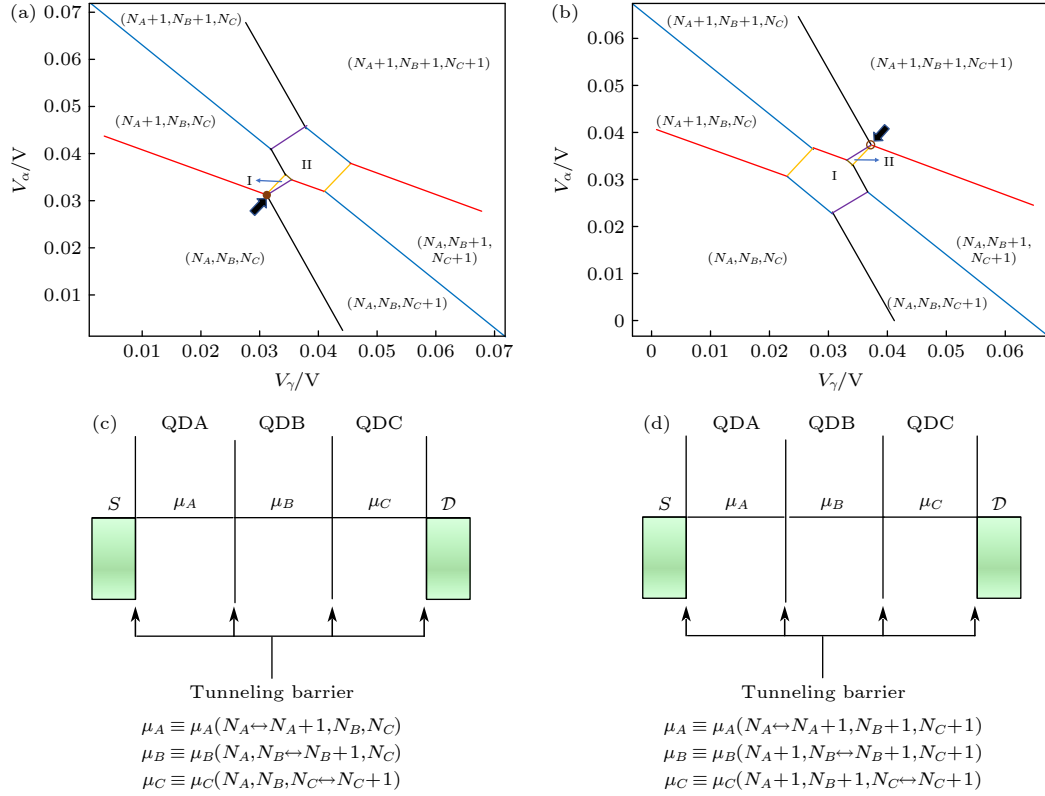
图 7 第一类四点, 其中 I 区指代的是 (N_A, N_B + 1, N_C) 区域, II 区指代的是 (N_A + 1, N_B, N_C + 1) 区域 (a) 在 V_\beta = 0.0109 V 下的二维稳态图. 箭头指代的实心点对应了电子运输的四点; (b) V_\beta = 0.0166 V. 箭头指代的空心点对应了空穴运输的四点. 图 (b) 对应二维稳态图的 V_\beta 值大于图 (a) 的 V_\beta 值; (c) 图 (a) 棕色实心点对应的电化学势对齐情况, QDA, QDB 和 QDC 分别指代的是量子点 A, B 和 C; (d) 图 (b) 棕色空心点对应的电化学势对齐情况, QDA, QDB 和 QDC 分别指代的是量子点 A, B 和 C
