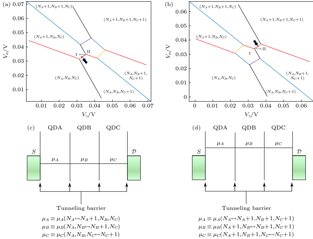
图 6 第三类三点, 其中 I 区指代的是 (N_A, N_B + 1, N_C) 区域, II 区指代的是 (N_A + 1, N_B, N_C + 1) 区域 (a) 对应了图 3 中的红色虚线方框, 这里 V_\beta = 0.0106 V. 箭头指代的实心点标示了在该三点处是电子型输运; (b) V_\beta = 0.0167 V. 箭头指代的空心点标示了在该三点处是空穴型输运. 图 (b) 对应二维稳态图的 V_\beta 值大于图 (a) 的 V_\beta 值; (c) 图 (a) 红色实心点对应的电化学势对齐情况, QDA, QDB 和 QDC 分别指代的是量子点 A, B 和 C. (d) 图 (b) 红色空心点对应的电化学势对齐情况, QDA, QDB 和 QDC 分别指代的是量子点 A, B 和 C
