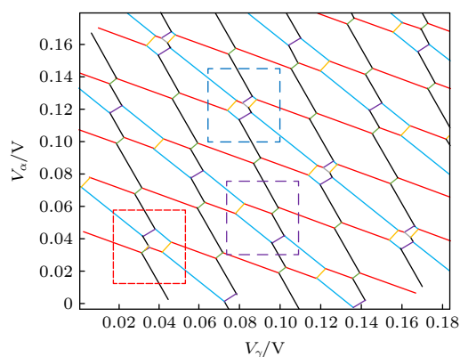
图 3 在中间量子点栅压 V_\beta = 0.0106 V 时的 STQD 的二维稳态图. 其中红色线、蓝色线和黑色线分别代表了量子点 A 、 B 、 C 的充电线; 黄色线、紫色线以及绿色线分别代表了电荷在量子点 A 和 B 、量子点 B 和 C 以及量子点 A 和 C 之间的电荷重分布线; 灰色线代表了 STQD 点独有的输运过程
