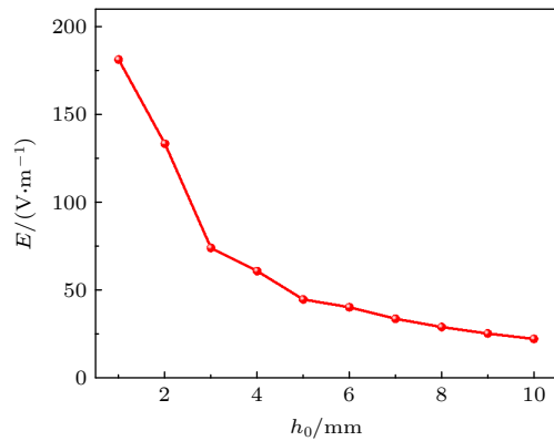
图 7 观测点电场强度随平行板间距的变化
