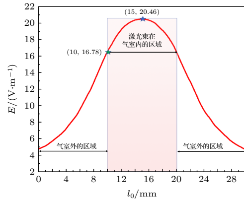
图 6 激光束路径上的电场强度
