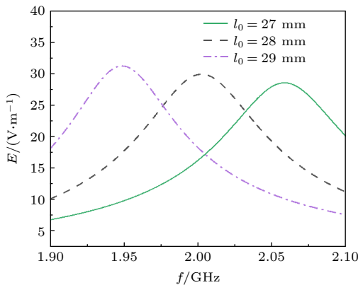
图 4 不同 PPTLR 长度 l_0 时, 观测点电场强度随频率的变化
