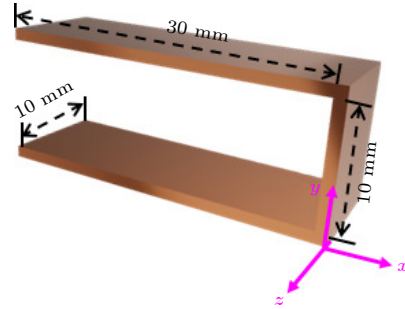
图 1 PPTLR 电场局域增强结构仿真示意图 Fig. 1. PPTLR electric field local enhancement structure simulation.
