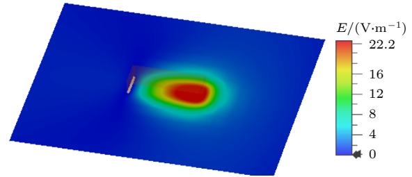
图 5 电场分布
