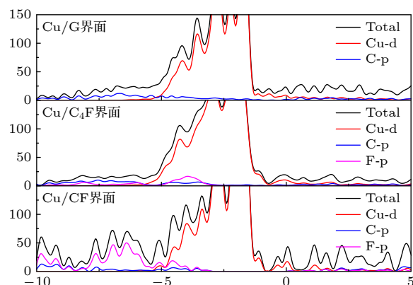
图 11 Cu/G、Cu/C 4 F 和 Cu/CF 界面的 DOS 图, 虚线为费米能级
