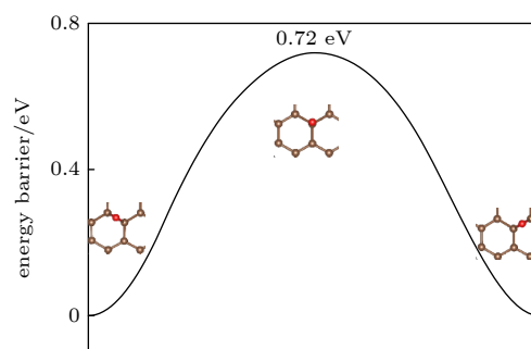
图3 O 原子在 G 相邻桥位上的扩散的能垒图
