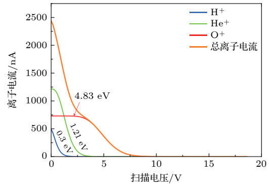
图 6 阻滞势分析仪伏安特性曲线
