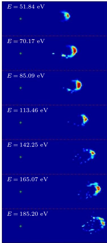
图 12 离子成像仪对 7 种能量离子的测试图像 (图中绿色星号为视场中心) Fig. 12. Images of 7 kinds of energy ions (the green asterisk is the center of the field view).
