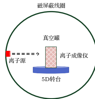
图 11 定标测试系统组成框图.
