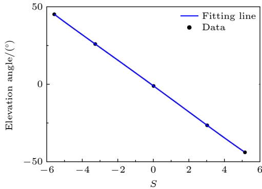
图 15 离子成像仪俯仰角与偏转板因子拟合曲线
