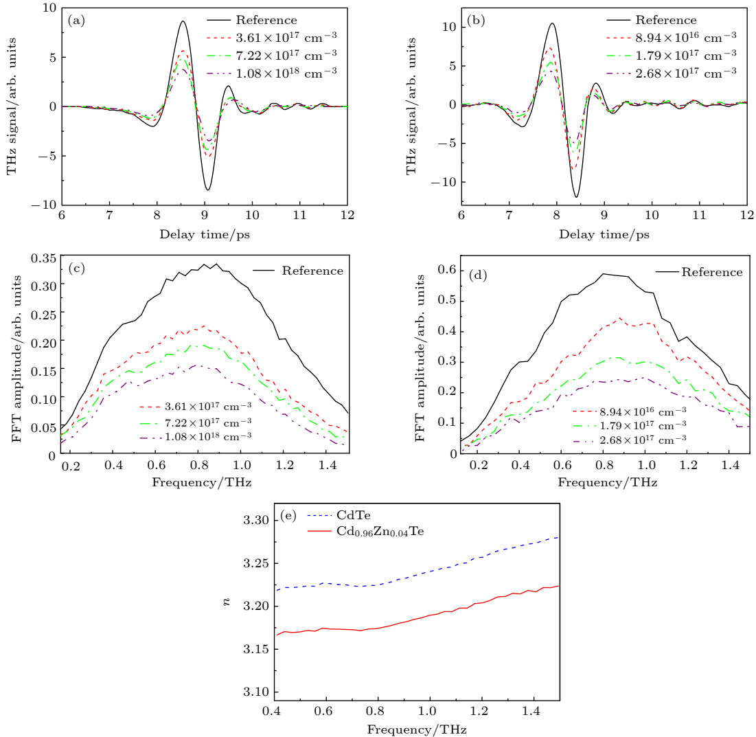
图 4 不同光激发载流子浓度下 \text{Cd}_{0.96}\text{Zn}_{0.04}\text{Te} (a) 和 \text{CdTe} (b) 的 THz 时域谱; 傅里叶变换后不同光激发载流子浓度下的 \text{Cd}_{0.96}\text{Zn}_{0.04}\text{Te} (c) 和 \text{CdTe} (d) 的频谱图; (e) 无抽运光激发时 \text{Cd}_{0.96}\text{Zn}_{0.04}\text{Te} 和 \text{CdTe} 的折射率图
