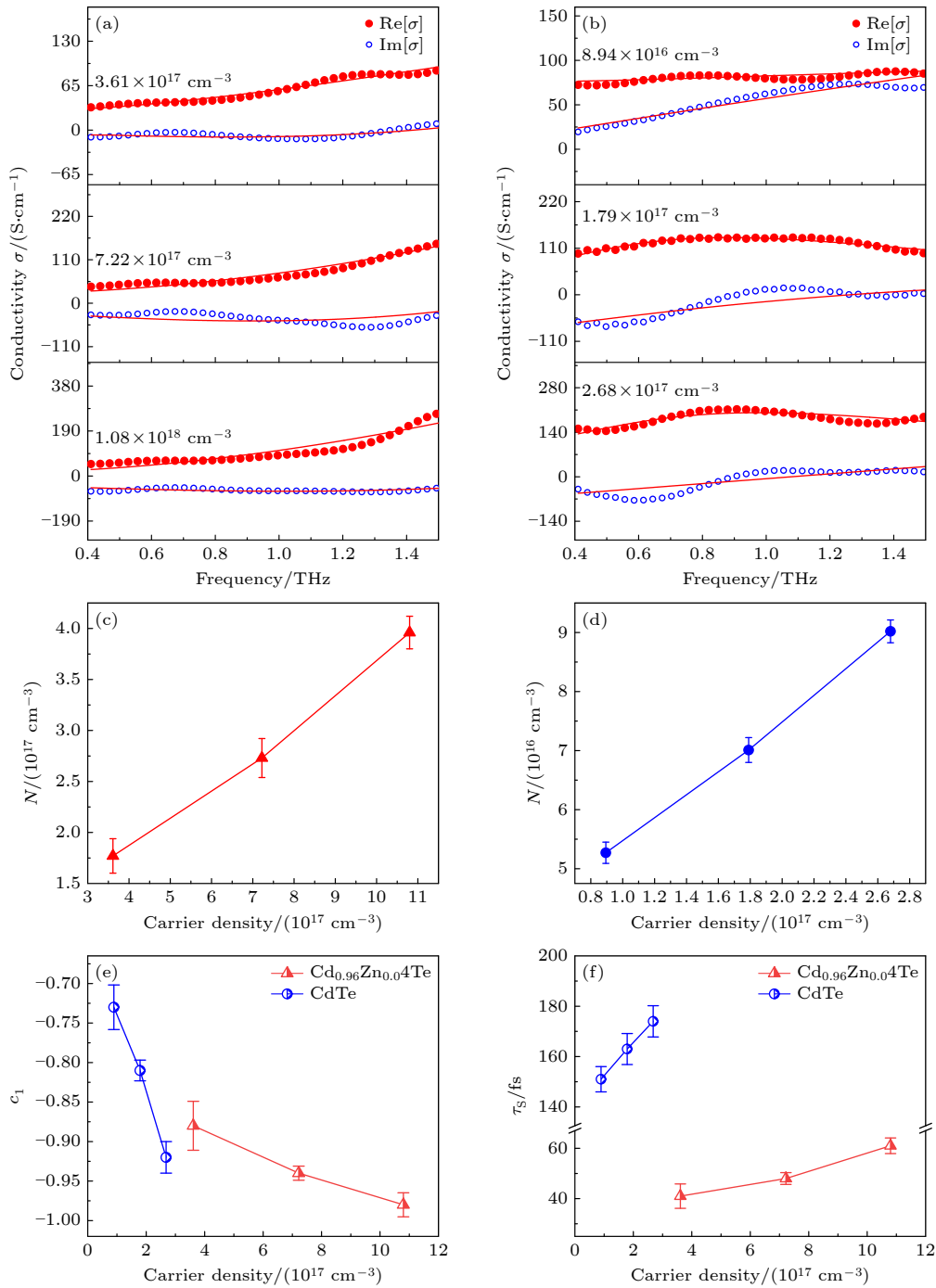
图 5 不同光激发载流子浓度下 Cd 0.96 Zn 0.04 Te (a) 和 CdTe (b) 的瞬态电导率, 实线为 Drude-Smith 模型的拟合结果; 延迟时间为 50 ps 时 Cd 0.96 Zn 0.04 Te (c) 和 CdTe (d) 的载流子浓度随光激发载流子浓度的变化关系; (e) Cd 0.96 Zn 0.04 Te (红) 和 CdTe (蓝) 的 Smith 参数 c_1 随光激发载流子浓度的变化关系图; (f) Cd 0.96 Zn 0.04 Te (红) 和 CdTe (蓝) 的载流子散射时间 \tau_s 随光激发载流子浓度的变化关系图
