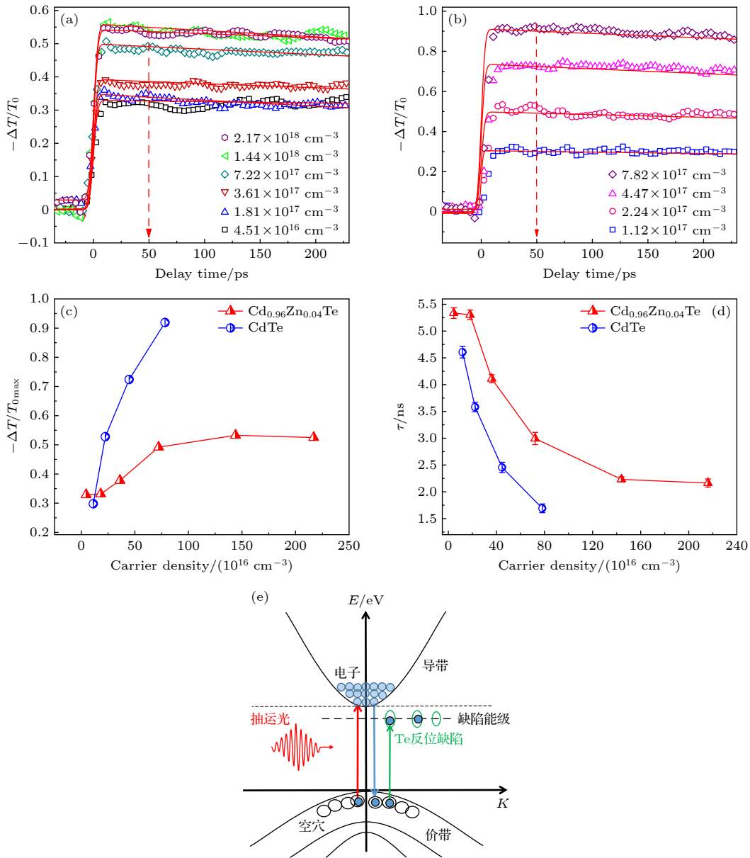
图 3 不同光激发载流子浓度下 \text{Cd}_{0.96}\text{Zn}_{0.04}\text{Te} (a) 和 \text{CdTe} (b) 的 THz 瞬态透射变化率与延迟时间的关系图, 实线是单指数函数拟合结果; (c) \text{Cd}_{0.96}\text{Zn}_{0.04}\text{Te} 和 \text{CdTe} 的 THz 瞬态透射变化率最大值 ( -\Delta T/T_{0\max} ) 与光激发载流子浓度的关系图; (d) \text{Cd}_{0.96}\text{Zn}_{0.04}\text{Te} 和 \text{CdTe} 的载流子复合时间与光激发载流子浓度的关系图; (e) \text{Cd}_{0.96}\text{Zn}_{0.04}\text{Te} 的能带结构示意图
