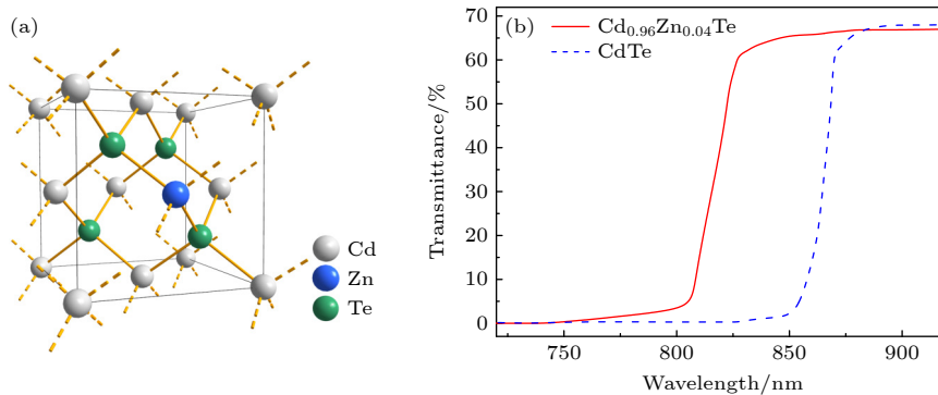
图 2 (a) Cd 0.96 Zn 0.04 Te 的晶体结构示意图; (b) Cd 0.96 Zn 0.04 Te (红) 和 CdTe (蓝) 室温下的紫外-可见透射光谱
