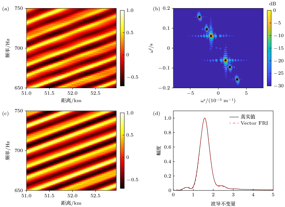
图 4 背景声速剖面干涉条纹的稀疏表示 (a) 规则干涉条纹 (无内波); (b) 干涉条纹的二维频谱 (背景图表示 2D-FFT 谱, 黑色方块表示 KRAKEN 计算的真实中心频率, 红色星号表示 vector-FRI 估计频率); (c) vector FRI 重建的干涉条纹; (d) 利用 2D-FFT 方法计算出的背景环境干涉条纹 (黑线) 和 vector FRI 恢复的干涉条纹 (红线) 对应的波导不变量分布
