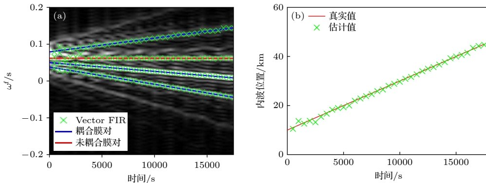
图 7 (a) 距离维频率 \omega^r = k_{12} 时, 频率维频率随时间的变化, 其中, 背景图表示傅里叶变换的结果, \times 表示 vector FRI 的估计结果, 红色直线表示由未耦合模对频率 (频率不随时间变化) 拟合的直线, 蓝色直线表示由耦合模对频率 (频率随时间变化) 拟合的直线; (b) 利用耦合模对频率估计出的内波轨迹
