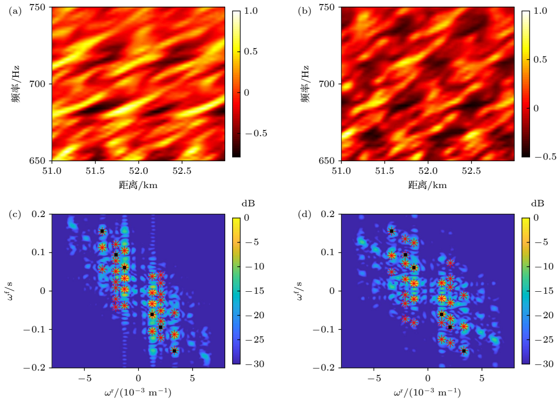
图 5 存在内波环境下干涉条纹图和对应的二维频谱图 (a) 和 (b) 分别表示内波位置距声源 24 km 和 35 km 处的干涉条纹图; (c) 和 (d) 分别表示 (a) 和 (b) 中干涉条纹的二维频谱图. 背景图表示 2D-FFT 谱, 黑色方块表示 KRAKEN 计算的真正中心频率, 红色星号表示 vector-FRI 估计频率
