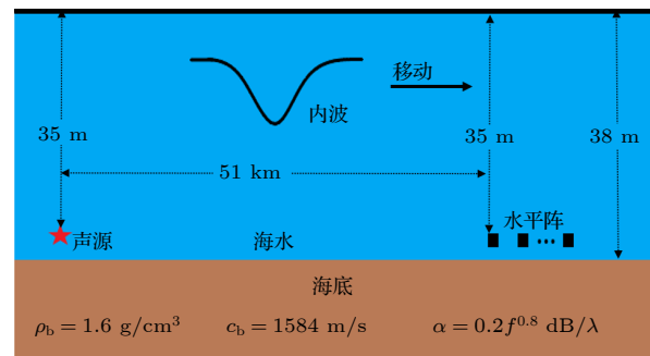
图 2 仿真设置示意图 Fig. 2. Diagram of simulation setting.
