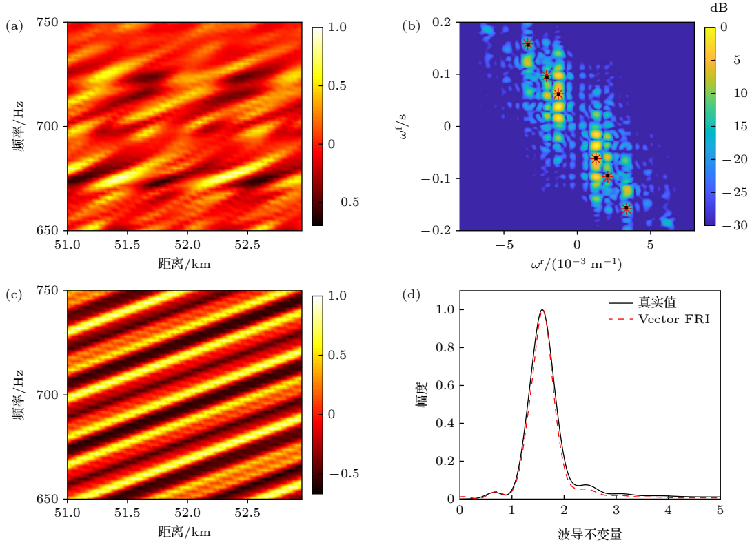
图 8 水下声场干涉条纹图的重构以及波导不变量的恢复; (a) 内波环境下 ( r_0 = 20 \text{ km} ) 的声场干涉条纹图; (b) 内波环境下 ( r_0 = 20 \text{ km} ) 声场干涉条纹图的二维傅里叶频谱, 背景图为 2DFFT 结果, 黑色方块表示 KRAKEN 计算的真正中心频率, 红色星号表示 vector-FRI 估计的未耦合模对频率; (c) 利用未耦合模对重建的干涉条纹图; (d) 波导不变量分布. 红线为内波环境下重建干涉条纹对应的波导不变量, 黑线为背景场 (无内波) 对应的波导不变量分布
