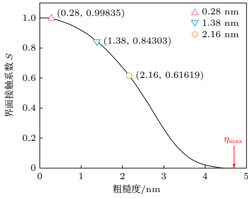
图4 界面接触系数 S 和粗糙度之间的关系, 其中 \eta_{\max} 为经验值, 是界面两侧材料的原子间经验势函数截止半径的10倍, 当界面粗糙度大于这个值时, 认为界面接触系数趋近于0, 对于 Al/Si 界面, 该值为 4.7 nm
