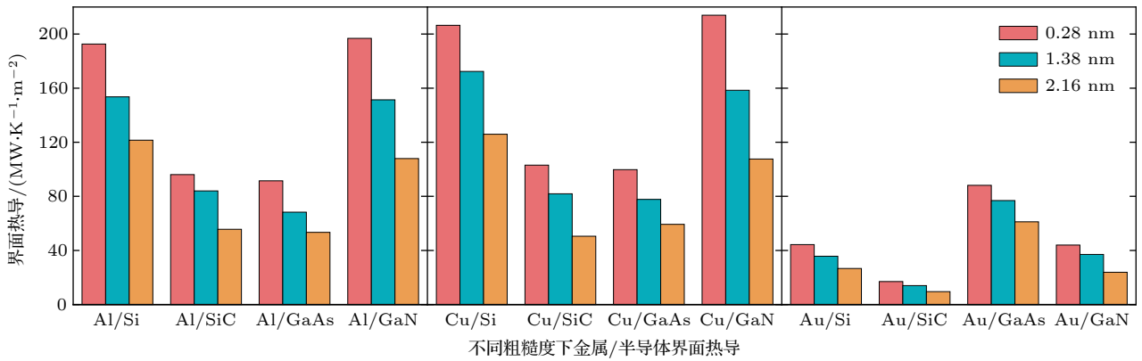
图 6 MMM 模型预测 300 K 时的金属 (Al, Cu, Au) 和半导体 (Si, SiC, GaAs, GaN) 界面热导, 其中粗糙度取值为 0.28, 1.38, 2.16 nm Fig. 6. Interfacial thermal conductance of metal (Al, Cu, Au) and semiconductor (Si, SiC, GaAs, GaN) interfaces predicted by MMM model at 300 K, roughness values: 0.28 nm, 1.38 nm, 2.16 nm.
