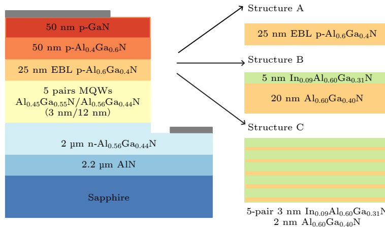
图 1 AlGa 0.4 N 基 DUV LED 结构示意图 (左) 和结构 A(单层 EBL)、B(双层 EBL)、C(超晶格结构 EBL)(右)
