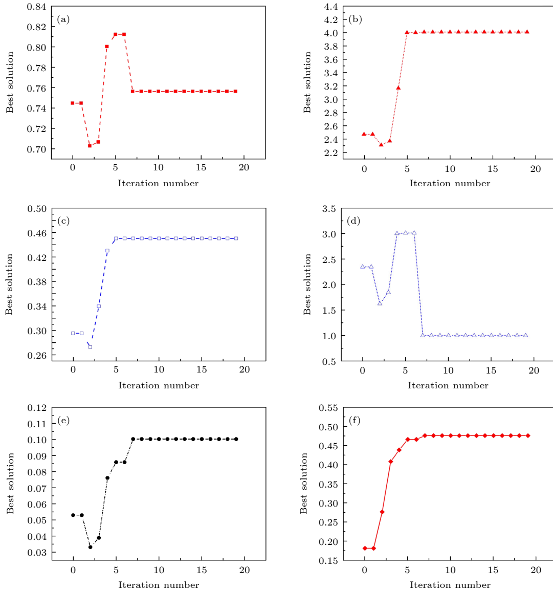
图4 InAlGa N /AlGa N 超晶格 EBL 结构参数和 IQE 随优化中迭代次数变化曲线: (a) 量子垒的 Al 组分 QB x ; (b) 量子垒的厚度 QB d ; (c) 量子阱的 Al 组分 QW x ; (d) 量子阱的厚度 QW d ; (e) 量子阱掺 In 的大小 y ; (f) 内量子效率 IQE
