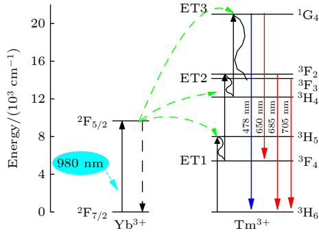
图 3 Yb^{3+} 敏化 Tm^{3+} 的上转换发光过程
