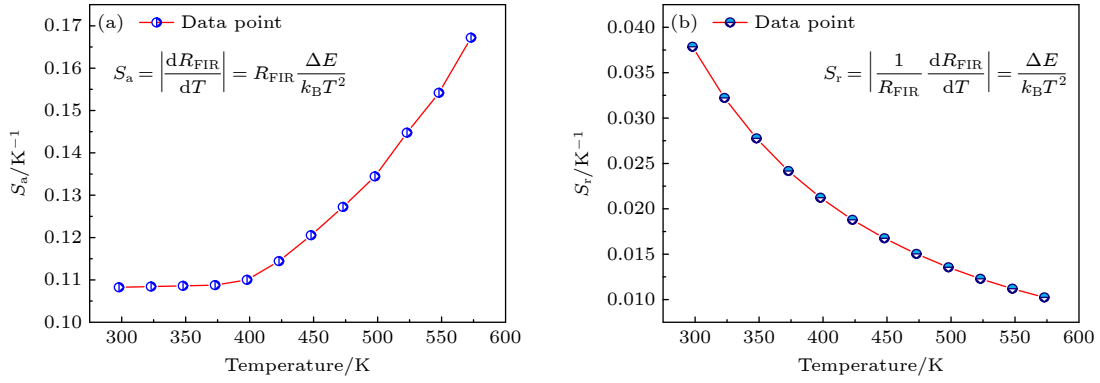
图 10 非热耦合能级对 {}^3F_3/{}^1G_4 表征温度时的绝对测温灵敏度 (a) 和相对测温灵敏度 (b)
