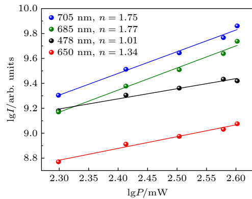
图 5 1% Tm^{3+} , 6% Yb^{3+}:Bi_2WO_6 的上转换发射强度与泵浦功率的关系
