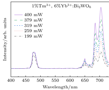
图 4 980 nm 激光激发下, 不同泵浦功率时 1% Tm^{3+} , 6% Yb^{3+}:Bi_2WO_6 的上转换光谱
