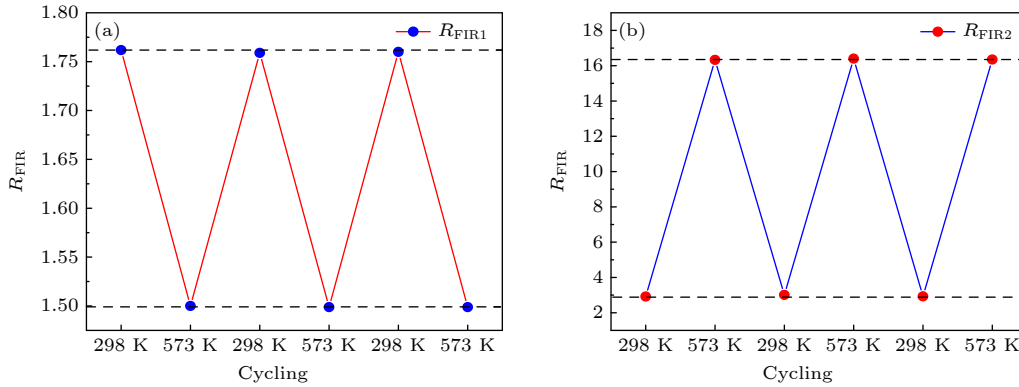
图 11 298 和 573 K 下 R_{FIR1} (a) 以及 R_{FIR2} (b) 稳定性测试
