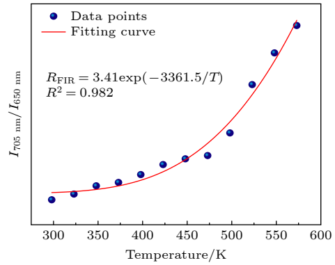
图 9 非热耦合能级对 {}^3\text{F}_3/{}^1\text{G}_4 产生的705和650 nm处荧光强度比与温度的关系
