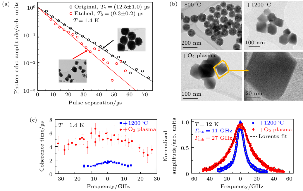
图 5 (a) 化学刻蚀前后 \text{Eu}^{3+}:\text{Y}_2\text{O}_3 纳米粉体的光学回波信号衰减曲线. 内附图为对应的纳米粉体的 TEM 形貌 [81] ; (b) \text{Eu}^{3+}:\text{Y}_2\text{O}_3 纳米粉体在初次 800 °C 煅烧 (左上), 二次 1200 °C 煅烧 (右上) 并微波等离子体处理后 (下) 的 TEM 形貌 [82] ; (c) \text{Eu}^{3+} 离子 ^5\text{D}_0-^7\text{F}_0 跃迁在不同制备条件下的光学相干时间 T_2 和非均匀线宽 \Gamma_{\text{inh}} . 样品在 0 处的光学跃迁频率为 (516.0979 \pm 0.0002) \text{ THz} ( (580.8830 \pm 0.0001) \text{ nm} ) [82]
