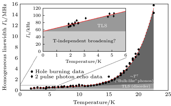
图 6 \text{Eu}^{3+}:\text{Y}_2\text{O}_3 纳米粉体的均匀线宽随温度的变化. 黑色、灰色和浅灰色区域分别表示双声子拉曼效应 (TPR)、局域无序二能级系统 (TSL) 以及与温度无关的光谱展宽的贡献. 在主图和插图中, 阴影区域都代表了与温度无关的展宽 (最浅)、TLS 相互作用展宽和 TPR 相互作用展宽 (最暗) [92]
