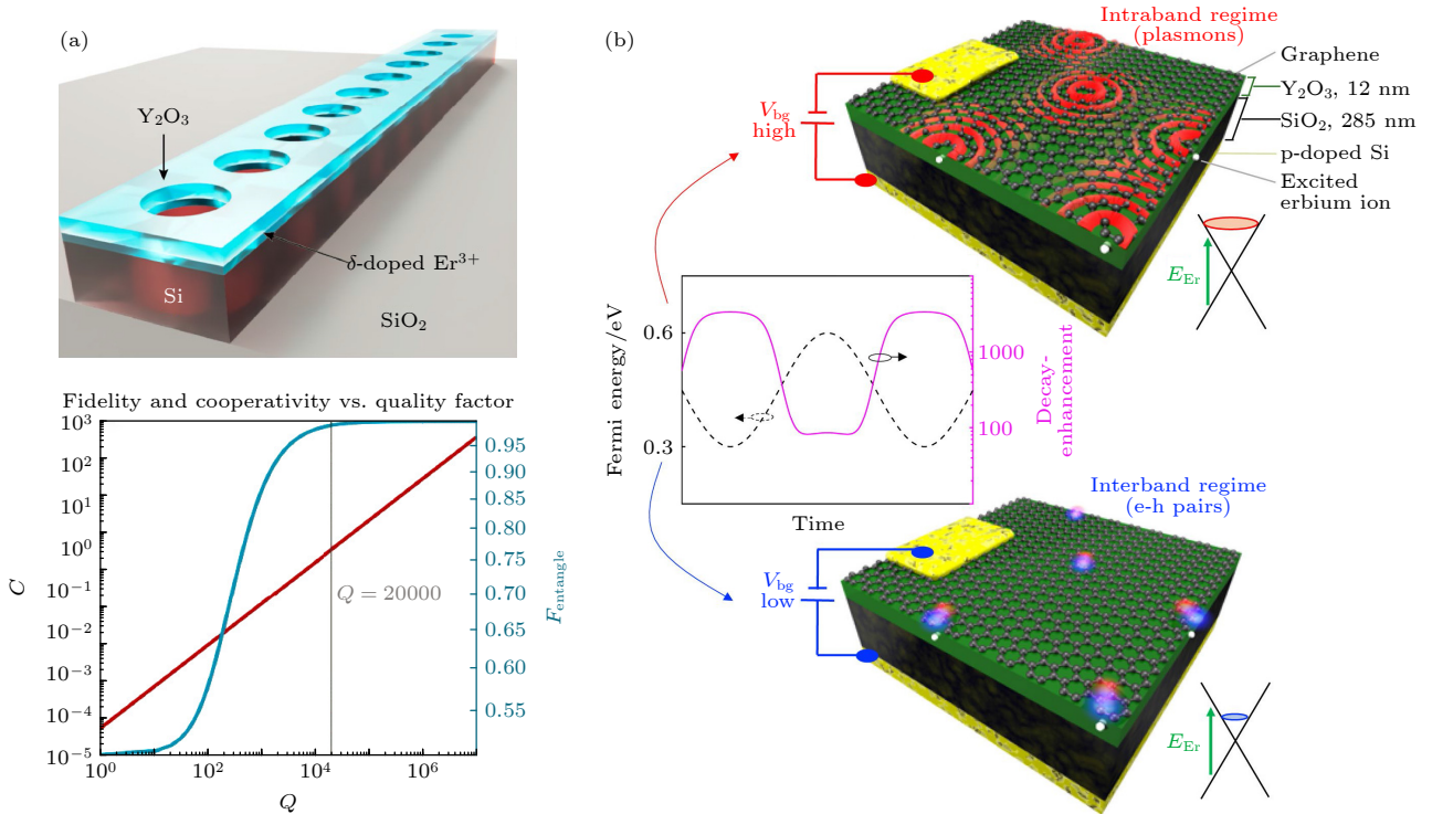
图9 (a) \text{Er}^{3+}:\text{Y}_2\text{O}_3 - \text{Si} 光子晶体腔结构示意图以及离子腔耦合协同性和纠缠保真度随腔质量因子的变化 [103] ; (b) \text{Er}^{3+}:\text{Y}_2\text{O}_3 -石墨烯杂化系统的动态调制示意图 [104]
