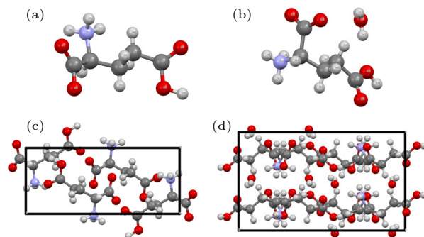
图 1 DL-Glu 及 DL-Glu·H 2 O 的分子结构 (a), (b) 及晶胞结构 (c), (d)
