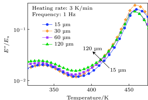
图 7 不同应变下 (\text{La}_{0.6}\text{Ce}_{0.4})_{65}\text{Al}_{10}\text{Co}_{25} 非晶合金归一化损耗模量 E''/E_u 随温度演化 (升温速率为 3 \text{ K/min} )
