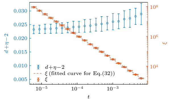
图 13 在 T > T_c 时, 不同约化温度 t 下关联长度 \xi 与指数 d + \eta - 2 的拟合结果. 其中蓝色的圈表示 d + \eta - 2 的拟合结果, 红色的星号表示 \xi 的拟合结果, 红色的虚线表示对 (32) 式进行拟合的结果. 其中横轴 t 和纵轴 \xi 采用了双对数坐标. 误差棒表示拟合参数置信度为 95% 的置信区间
