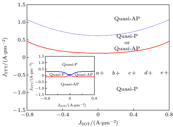
图 2 以自旋转移矩电流密度 J_{STT} 和自旋轨道矩电流密度 J_{SOT} 为控制参数的相图 (外磁场 h_0 = 2 ), 插图 h_0 = 0 时的磁性状态相图
