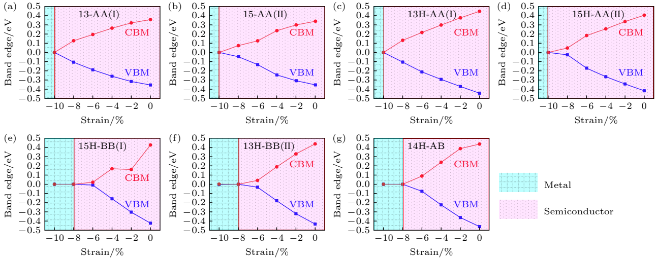
图 7 C_3B 纳米带带边 (CBM 及 VBM) 随应变变化 (a) 13-AA(I); (b) 15-AA(II); (c) 13H-AA(I); (d) 15H-AA(II); (e) 15H-BB(I); (f) 13AH-BB(II); (g) 14H-AB
