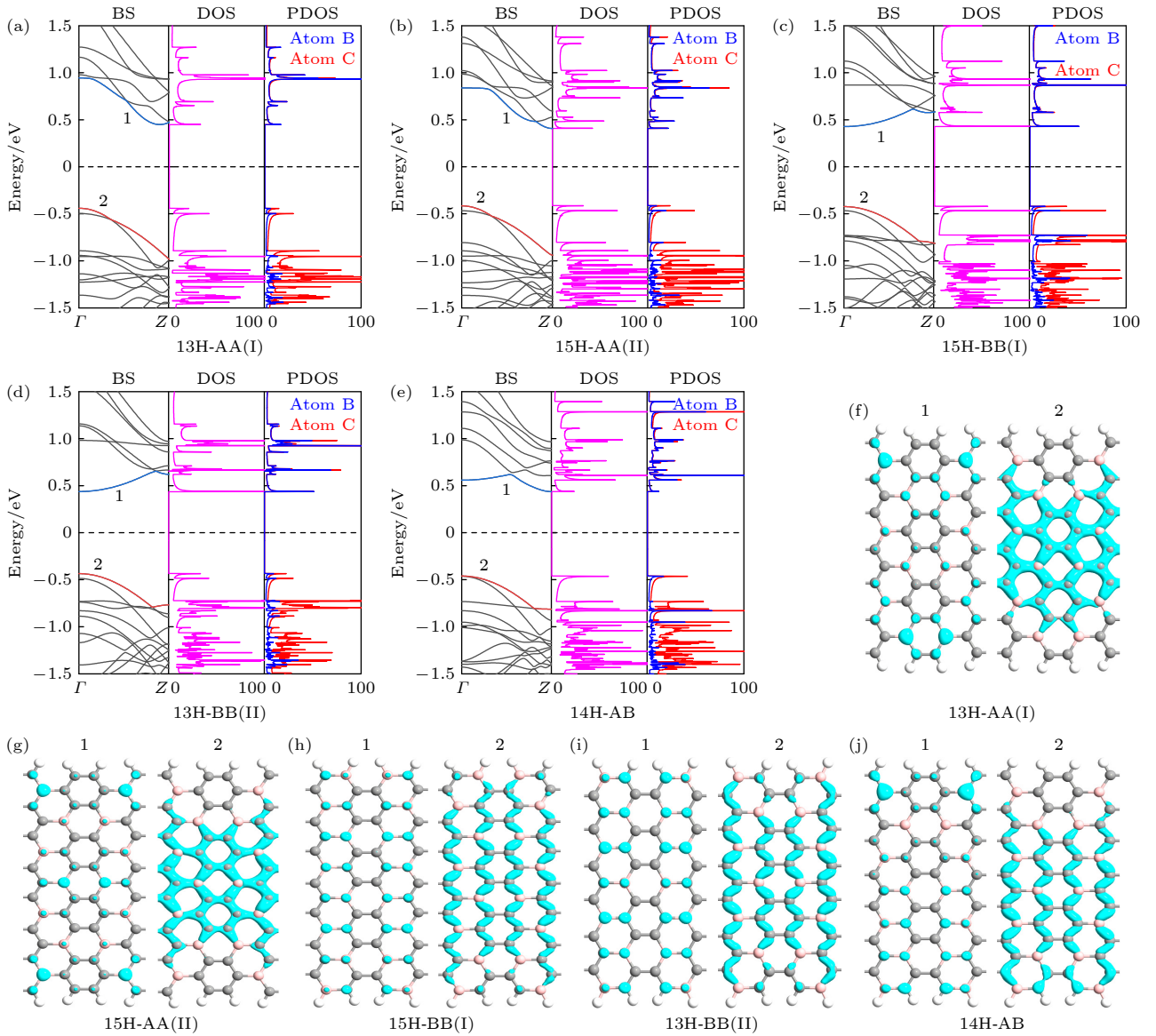
图 4 几种典型的 H 端接的 C_3B 纳米带的能带结构, 态密度 (DOS) 和原子投影态密度 (PDOS) (a) 13H-AA(I), (b) 15H-AA(II), (c) 15H-BB(I), (d) 13H-AA-BB(II), (e) 14H-AB; 相对应纳米带的能带 1 和 2 的部分电荷密度: (f) 13H-AA(I), (g) 15H-AA(II), (h) 15H-BB(I), (i) 13H-AA-BB(II), (j) 14H-AB, 部分电荷密度等值设为 0.03 |e| \cdot \text{\AA}^{-3}
