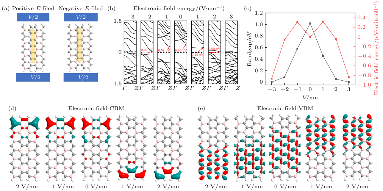
图 8 (a) 14H-AB 纳米带的电场调控效应; (b) 能带结构随电场变化; (c) 带隙及电场能随电场变化; (d), (e) CBM 和 VBM 的布洛赫态随电场变化, 布洛赫态等值面为 0.1 |e| \cdot \text{\AA}^{-3}
