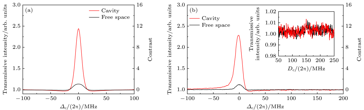
图 2 探测光在穿过自由空间的原子介质 (黑线) 和通过内置有原子介质的腔 (红线) 的透射强度 (左轴) 和光谱的对比度 (右轴) 随耦合光失谐变化的理论 (a) 和实验 (b) 结果. 实验和理论有相同的参数 \Omega_p/(2\pi) = 10 MHz, \Omega_c/(2\pi) = 14.4 MHz, \Gamma_c/(2\pi) = 5.2 MHz, \Gamma_l/(2\pi) = 1 MHz, N_a = 3 \times 10^{10} \text{ cm}^{-3} . 插图是将远失谐处的光谱放大来比较腔和自由空间光谱的噪声大小
