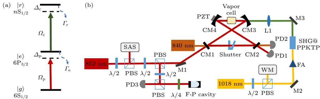
图1 (a) 铯 133 Cs原子里德伯态激发的阶梯型能级及耦合的激光. 其中 |g\rangle , |e\rangle 和 |r\rangle 分别表示铯原子基态、激发态和里德伯态, 852 nm的探测光和509 nm的耦合光分别耦合基态到激发态和激发态到里德伯态的跃迁, \Delta_p 和 \Delta_c 分别为探测光和耦合光的失谐, \Omega_p 和 \Omega_c 分别为探测光和耦合光的拉比频率, \Gamma_e 和 \Gamma_r 分别为激发态和里德伯态能级的衰减. (b) 铯原子里德伯原子光谱实验装置图. \lambda/2 , 半波片; \lambda/4 , 1/4波片; CM, 腔镜; M, 反射镜; L, 透镜; PD, 光电探测器; SAS, 饱和吸收光谱; PZT, 压电换能器; PBS, 偏振分束器; FA, 光纤功率放大器; SHG, 二次谐波产生; WM, 波长计; Shutter, 光开关; F-P cavity, 法布里-珀罗腔
