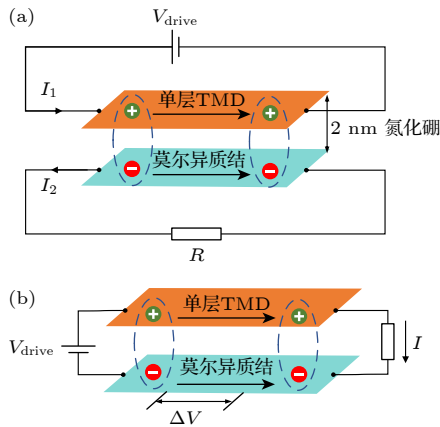
图6 激子电输运实验示意图 (a) 库仑拖拽实验: 单层 TMD 与莫尔异质结晶格之间有 2 nm 的氮化硼中间层, 单层 TMD 和莫尔异质结分别处于不同回路, 在单层 TMD 中施加电流 I_1 , 测量在莫尔异质结中的拖拽电流 I_2 , 这里莫尔异质结回路没有外加电流源, 激子形成宏观相干态后, I_1 = I_2 , 并且回流实验 (b) 观测到没有耗散的层内电流 ( \Delta V = 0 )
