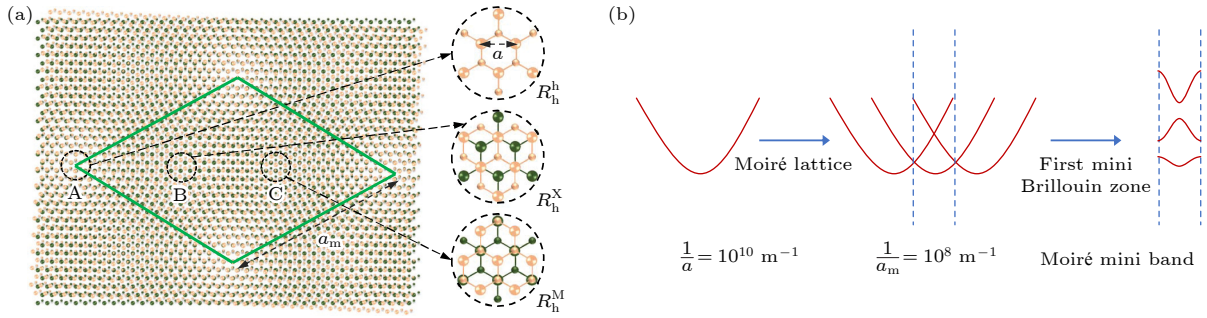
图 2 莫尔平带 (a) 在 TMD 异质结中形成的莫尔晶格 [25] , 其中 A, B, C 三个位置是莫尔格点中的高对称点, a_m 为莫尔周期, 其上下层原子堆叠情况参照右边的放大示意图 (此图为转角 0^\circ 附近); (b) 在形成莫尔晶格后, 布里渊区从原来的 1/a ( 10^{10} \text{ m}^{-1} ) ( a 为原子间距) 折叠为 1/a_m ( 10^8 \text{ m}^{-1} ), 形成迷你布里渊区, 在其边界通过布拉格反射打开能隙, 形成莫尔平带
