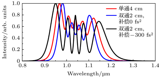
图 3 15 nJ, 100 fs 输入脉冲在光纤末端产生的输出光谱. 其中红线、蓝线和黑线分别对应单通 4 cm 光纤; 通过 2 cm 光纤后假定脉冲能量损耗 50% 后, 第二次经过 2 cm 光纤; 通过 2 cm 光纤后假定脉冲能量损耗 50% 以及补偿 -300 fs 2 色散后, 第二次经过 2 cm 光纤
