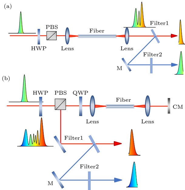
图 1 (a) 单通 SESS 与 (b) 色散管理双通 SESS 装置示意图 (PBS, 偏振光束分束器; Lens, 光学透镜; HWP, 半波片; QWP, 1/4 波片; CM, 啁啾镜; M, 反射镜)
