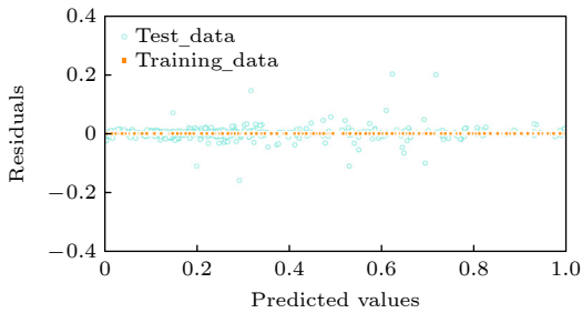
图3 标准情况决策树模型残差图
