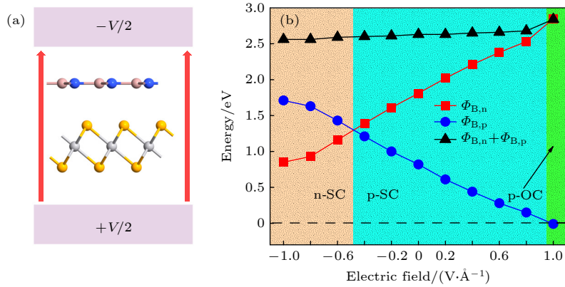
图 6 外加电场效应 (a) 异质结 S1 施加外电场作用示意图; (b) 异质结的肖特基势垒高度 \Phi_{B,n} , \Phi_{B,p} 和 GaN 单层的带隙 E_g 随电场的变化
