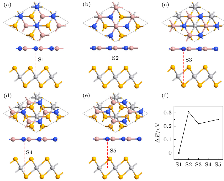
图2 GaN与1T-VSe 2 单层形成异质结时不同堆叠方式, GaN层的N原子分别对齐1T-VSe 2 层的(a) V原子, (b) 上层Se原子, (c) 下层Se原子, (d) V-Se键中间, 以及(e) 空位, 并记为S1—S5. (f) 5种堆叠方式的最低能量的相对值 \Delta E
