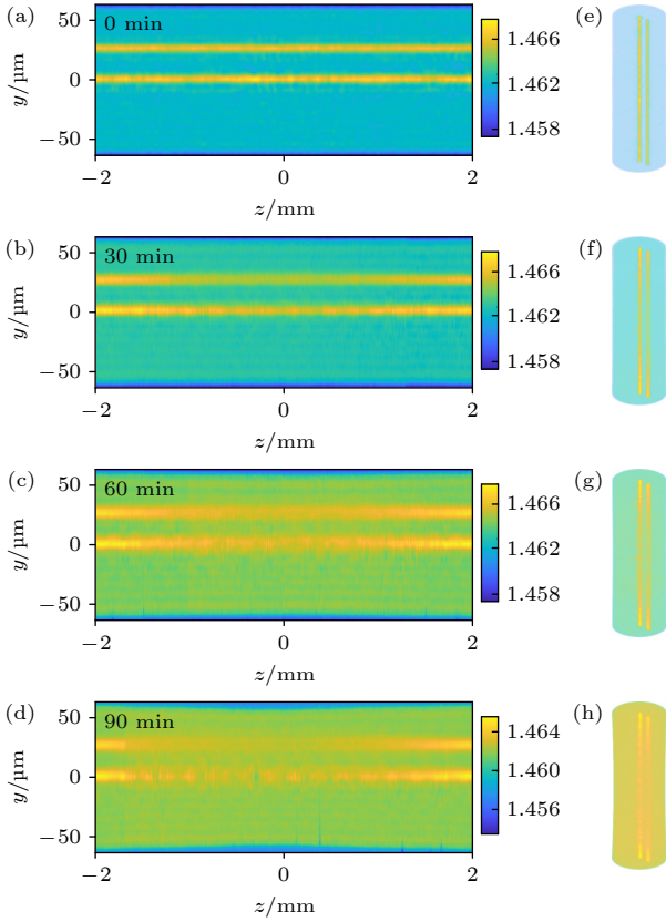
图4 加热时间分别为 (a) 0, (b) 30, (c) 60, (d) 90 min 时, 双芯光纤热扩散区 y - z 方向的折射率分布; 加热时间分别为 (e) 0, (f) 30, (g) 60, (h) 90 min 时, 双芯光纤热扩散区的三维折射率分布
