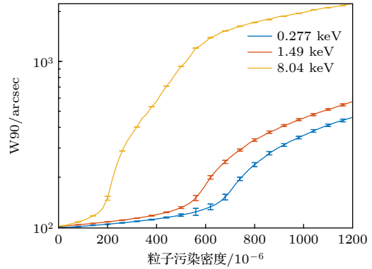
图 18 QM 件的 W90 随污染物密度变化关系
