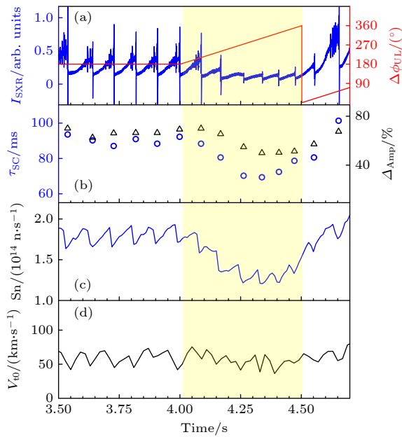
图 5 EAST #116507 炮放中等离子体参数的演变 (a) 芯部 SXR 辐射信号 (蓝色) 和 RMP 上下线圈相位差 (红色); (b) 锯齿周期 (蓝色圆圈) 和崩塌幅度 (黑色三角); (c) 中子产额; (d) 等离子体芯部旋转速度
