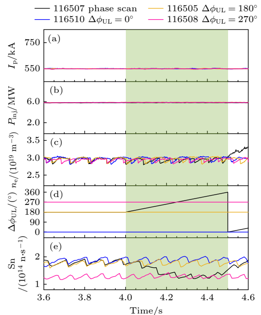
图 6 I_{RMP} = 3.5 kA 时, EAST 四炮等离子体参数的演变 (a) 等离子体电流; (b) 中性束注入功率; (c) 等离子体密度; (d) n = 2 的 RMP 上下线圈相位差; (e) 中子产额
