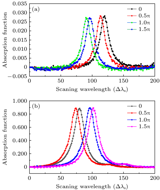
图 8 在两种测量中, 从对应的数据矩阵中选择不同波长调制相位处的数据切片轮廓所得到的气体吸收函数轮廓 (a) CO; (b) CO 2
