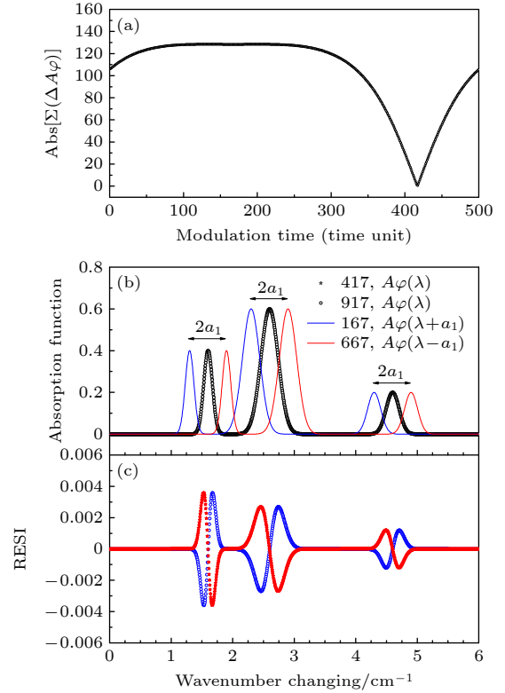
图 2 (a) 对应的两个间隔半个周期的吸收函数面积绝对值之差随调制时间的演化曲线; (b) 两个标准吸收函数曲线和调制时间偏移 1/4 周期对应的吸收函数曲线; (c) 图 (b) 中的两个标准吸收函数曲线和理论值的残值误差
