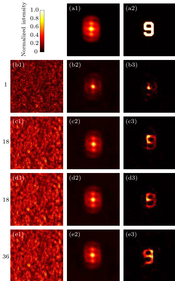
图 4 偏振复用散射相关成像 (a1), (b2), (c2), (d2), (e2) 自相关; (a2) 物体; (b1), (c1), (d1), (e1) 散斑图案; (b3), (c3), (d3), (e3) 重建图案
