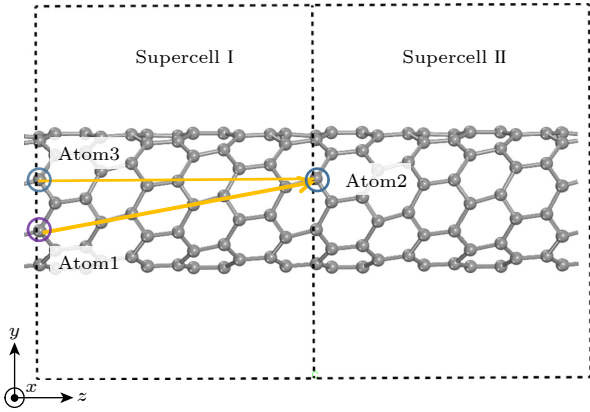
图 3 (8, 0) 单壁碳纳米管扭转后模型图 (扭转强度 = 3.52 (°)/Å)
