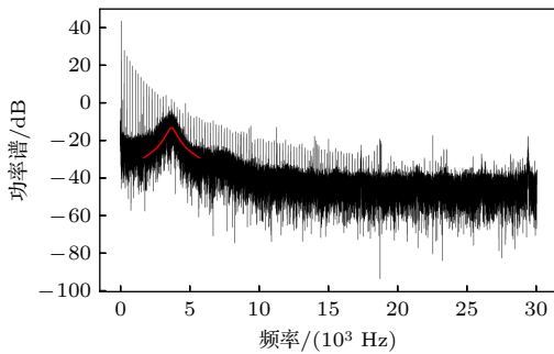
图 7 添加滤光片之后激光反馈实验信号功率谱示例
