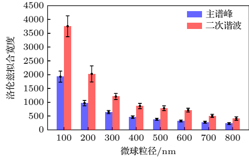
图 8 不同粒径激光反馈信号功率谱的洛伦兹宽度
