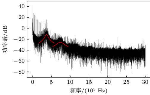
图 6 激光反馈实验信号功率谱示例
