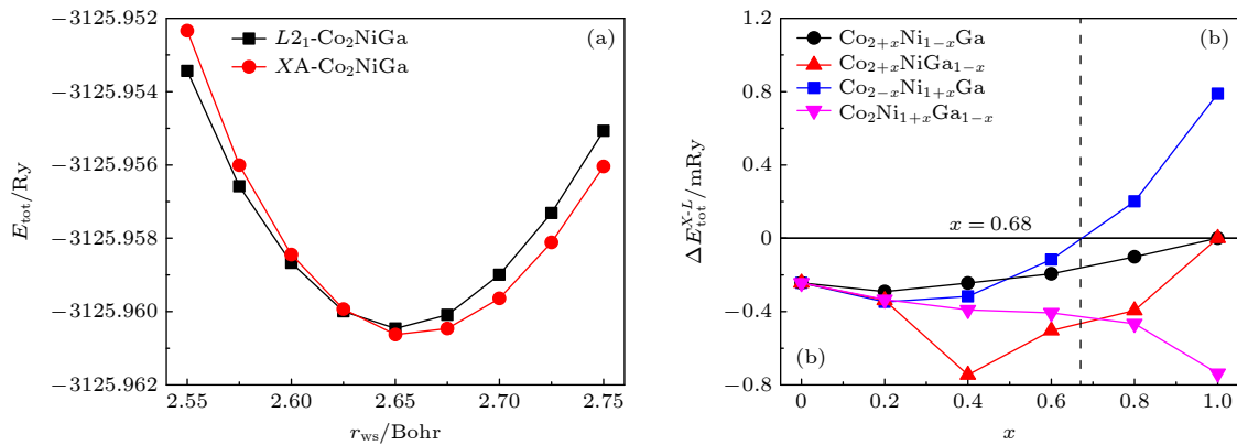
图 2 L2_1 -和 \text{XA-Co}_2\text{NiGa} 合金 E_{\text{tot}} 随 r_{\text{ws}} 的变化关系, 及四组非化学计量比合金平衡体积下 \Delta E_{\text{tot}}^{X-L-x} 关系 (a) E_{\text{tot}} ; (b) \Delta E_{\text{tot}}^{X-L}
