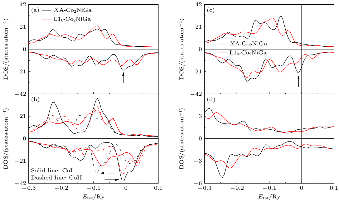
图 8 XA-和 L1_0 - \text{Co}_2\text{NiGa} 合金电子总态密度 (DOS), CoI 和 CoII, Ni, Ga 原子的局域 DOS 对比 (a) Tot; (b) CoI and CoII; (c) Ni; (d) Ga Fig. 8. Total electron density of states (DOS) and local DOS corresponding to CoI and CoII, Ni, Ga atoms of XA- and L1_0 - \text{Co}_2\text{NiGa} alloys: (a) Tot; (b) CoI and CoII; (c) Ni; (d) Ga.
