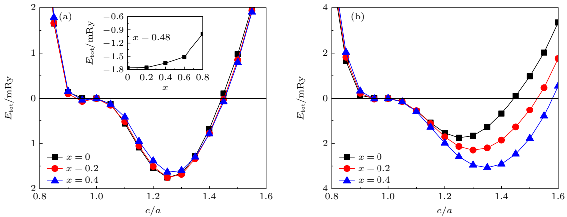
图 5 XA-Co_{2-x}Ni_{1+x}Ga 和 Co_2Ni_{1+x}Ga_{1-x} ( 0 \leq x \leq 0.4 ) 合金 E_{tot} 随 c/a 的变化关系 (a) Co_{2-x}Ni_{1+x}Ga ; (b) Co_2Ni_{1+x}Ga_{1-x}
