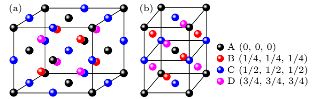
图 1 Co 2 NiGa 合金晶体结构图 (a) 奥氏体相; (b) 马氏体相
