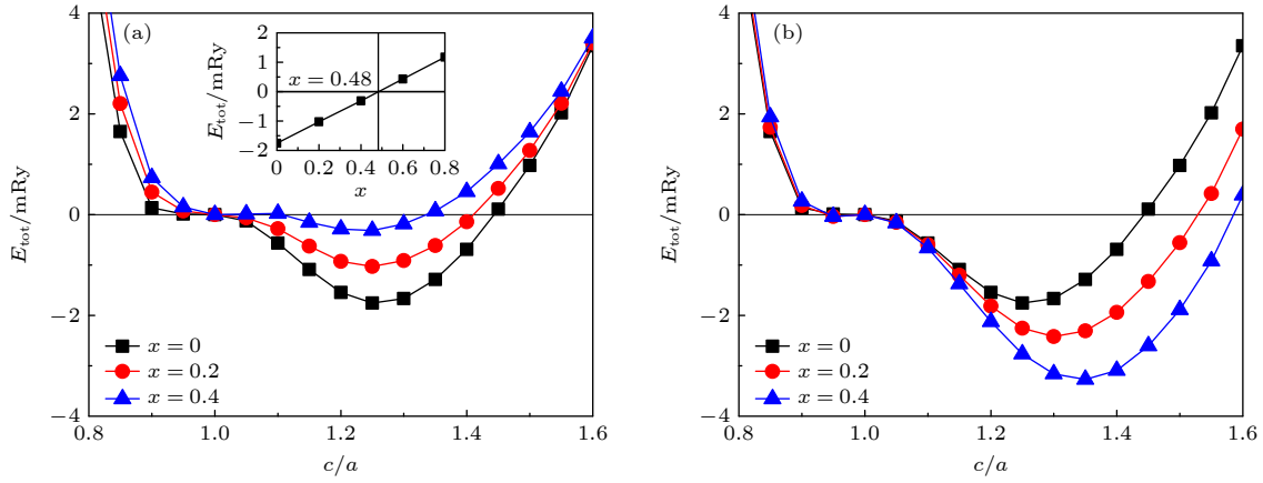
图 4 XA-Co_{2+x}Ni_{1-x}Ga 和 Co_{2+x}NiGa_{1-x} ( 0 \leq x \leq 0.4 ) 合金 E_{tot} 随 c/a 的变化关系 (a) Co_{2+x}Ni_{1-x}Ga ; (b) Co_{2+x}NiGa_{1-x}
