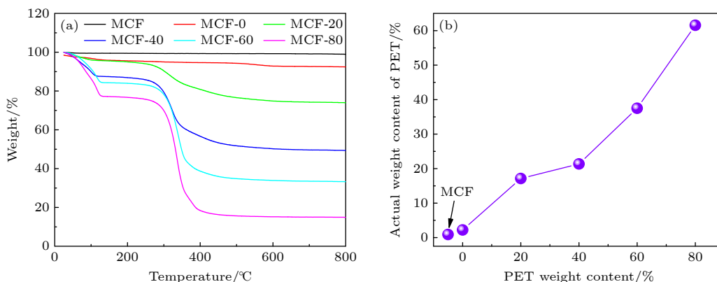
图 3 (a) 不同样品的 TGA 曲线; (b) 样品中的实际 PEI 含量 Fig. 3. (a) TGA curves of different samples; (b) actual PEI content in the studied samples.
