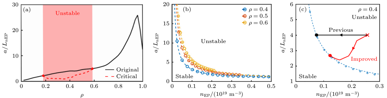
图 3 (a) 输运前的 AE 不稳定区间; (b) 在 \rho = 0.4, 0.5, 0.6 处, a/L_{\text{nEP}} 与 n_{\text{EP}} 的反比例关系; (c) \rho = 0.4 处, 旧模型和改进模型模拟的密度演化轨迹
