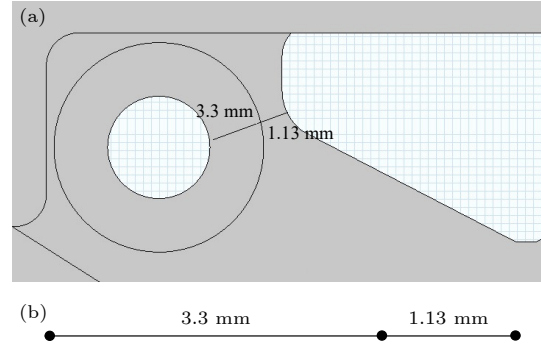
图 1 预电离的一维计算模型 Fig. 1. 1D model for preionization.
