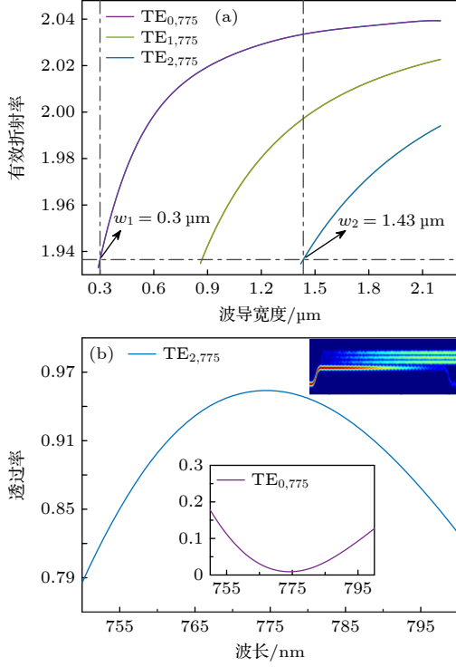
图 2 (a) 775 nm 泵浦光在 TE 0 , TE 1 , TE 2 模式下有效折射率随波导宽度的变化; (b) 非对称定向耦合器的自由光谱范围以及模拟光场分布图
