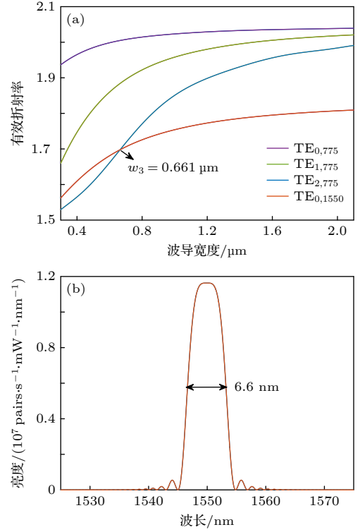
图 3 (a) 775 nm 的 TE 0 , TE 1 , TE 2 模式光和 1550 nm 的 TE 0 模式光的有效折射率随波导宽度的变化; (b) 输出参量光光谱图
