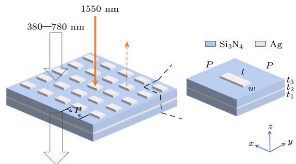
图 1 超表面减反射膜示意图
