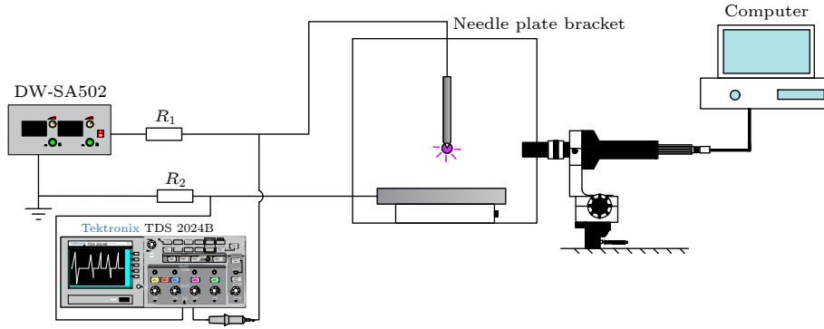
图 2 实验原理图
