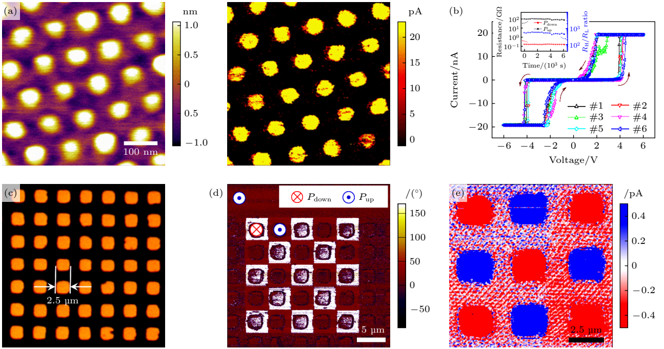
图3 铁电阻变与光伏效应 (a) Pt/BFO/SRO 纳米电容器阵列的形貌和导电原子力显微镜图像 [36] ; (b) Pt/BFO/SRO 纳米电容器的电流-电压多次循环回线, 左上为纳米电容器阻变开关比保持特性曲线 [36] ; (c) Au/Ti/T-BFO/LSMO 微米器件阵列的光学显微镜图像 [38] ; (d) Au/Ti/T-BFO/LSMO 微米器件阵列的 PFM 相位图, 其中亮区表示极化朝下, 暗区表示极化朝上 [38] ; (e) 导电原子力显微镜测得微米电极上的光电流图像 [38]
