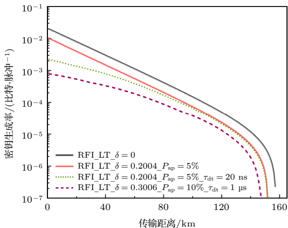
图4 基于不同设备缺陷的 RFI 协议以及 LT-RFI 协议密钥生成率图
