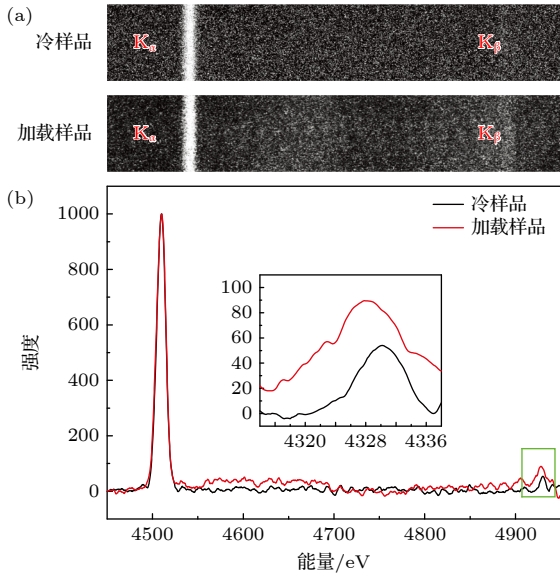
图 3 不同状态 Ti 样品的荧光光谱 (a) 原始图像; (b) 解谱结果
