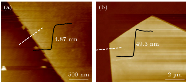
图 3 纳米片的 AFM 表征 (a) 薄纳米片 AFM 表征; (b) 厚纳米片 AFM 表征 Fig. 3. AFM characterization of nanosheets: (a) AFM characterisation of thin nanosheet; (b) AFM characterization of thick nanosheet.
