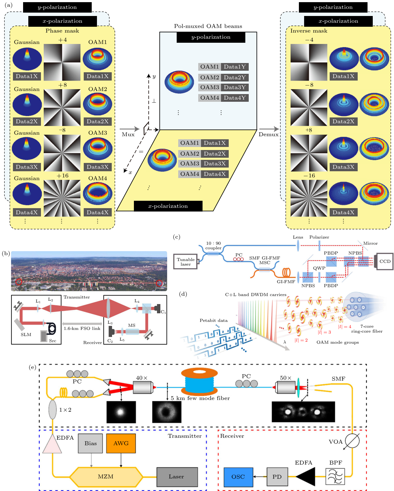
图 7 (a) 载有信息的涡旋光束的复用/解复用以及偏振复用/解复用 [98] ; (b) 埃尔朗根天际线 1.6 km 远的自由空间扭曲光路路径和实验装置图 [103] ; (c) 用于表征生成的涡旋光束的实验装置 [104] ; (d) OAM-SDM-WDM 数据传输的实验装置 [105] ; (e) OAM 复用光纤通信系统的实验装置, 实验装置包括发射器、OAM(解)复用器和接收器 [80]
