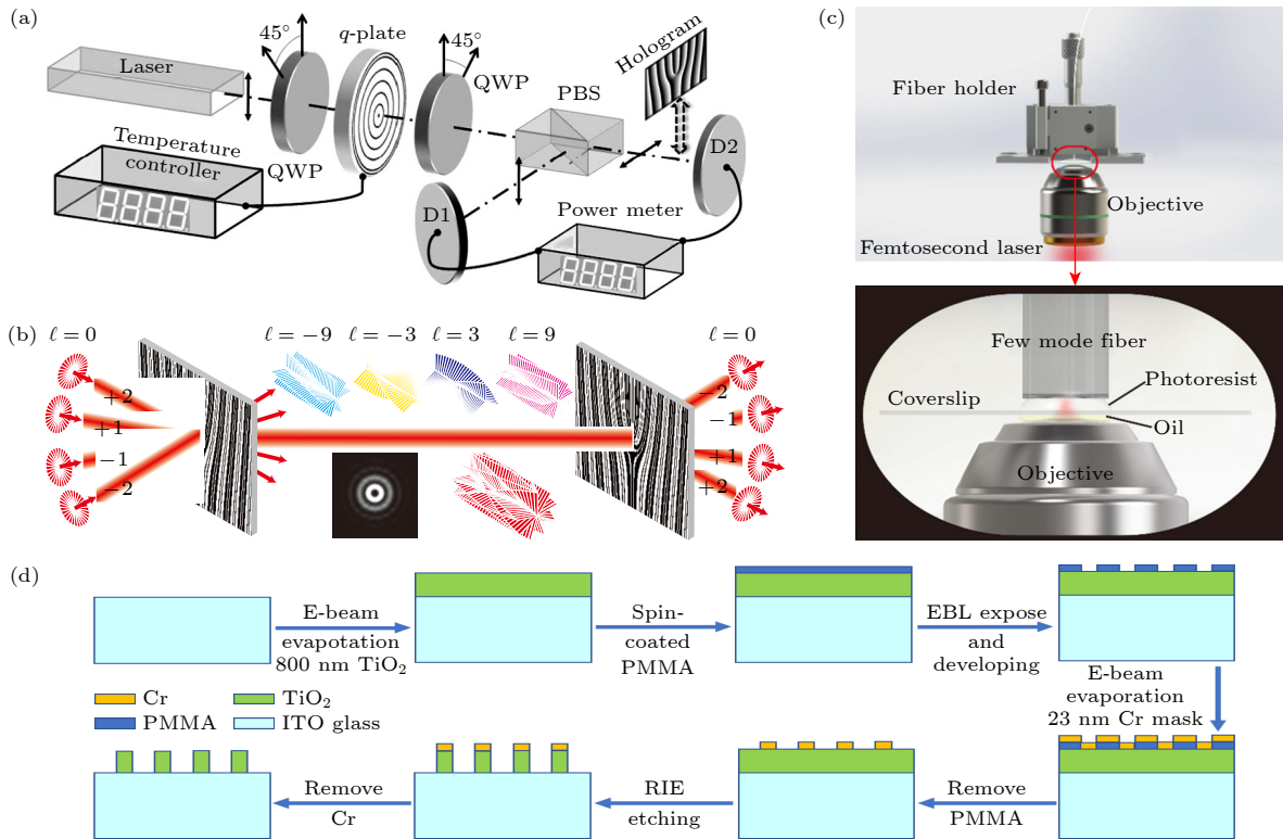
图 5 (a) 光子的 SAM 变化转换为 OAM 的装置示意图 [76] ; (b) 基于达曼光栅进行 OAM(解)复用的自由空间光通信示意图 [22] ; (c) 使用双光子光刻技术在少模光纤表面上制造涡旋光栅示意图 [80] ; (d) 基于电子束刻蚀法制作的超表面流程图 [81] Fig. 5. (a) The schematic of SAM-OAM mode converter [76] ; (b) the schematic of free-space optical communication based on Damann grating for OAM (de)multiplexing [22] ; (c) the details of fabricating vortex gratings on the surface of few-mode optical fibers using two-photon lithography [80] ; (d) flow chart of producing metasurface based on electron beam etching [81] .
