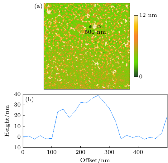
图 7 空气下疏水化基板表面 AFM 扫描结果 (a) 表面形貌; (b) 表面粗糙度扫描曲线
