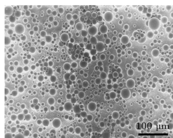
图 2 玻璃微球的 SEM 照片 Fig. 2. SEM photos of glass microspheres.
