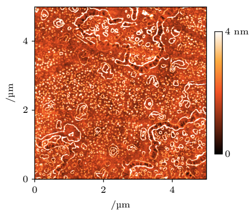
图 1 玻璃载玻片表面形貌图 Fig. 1. Surface topography of glass.
