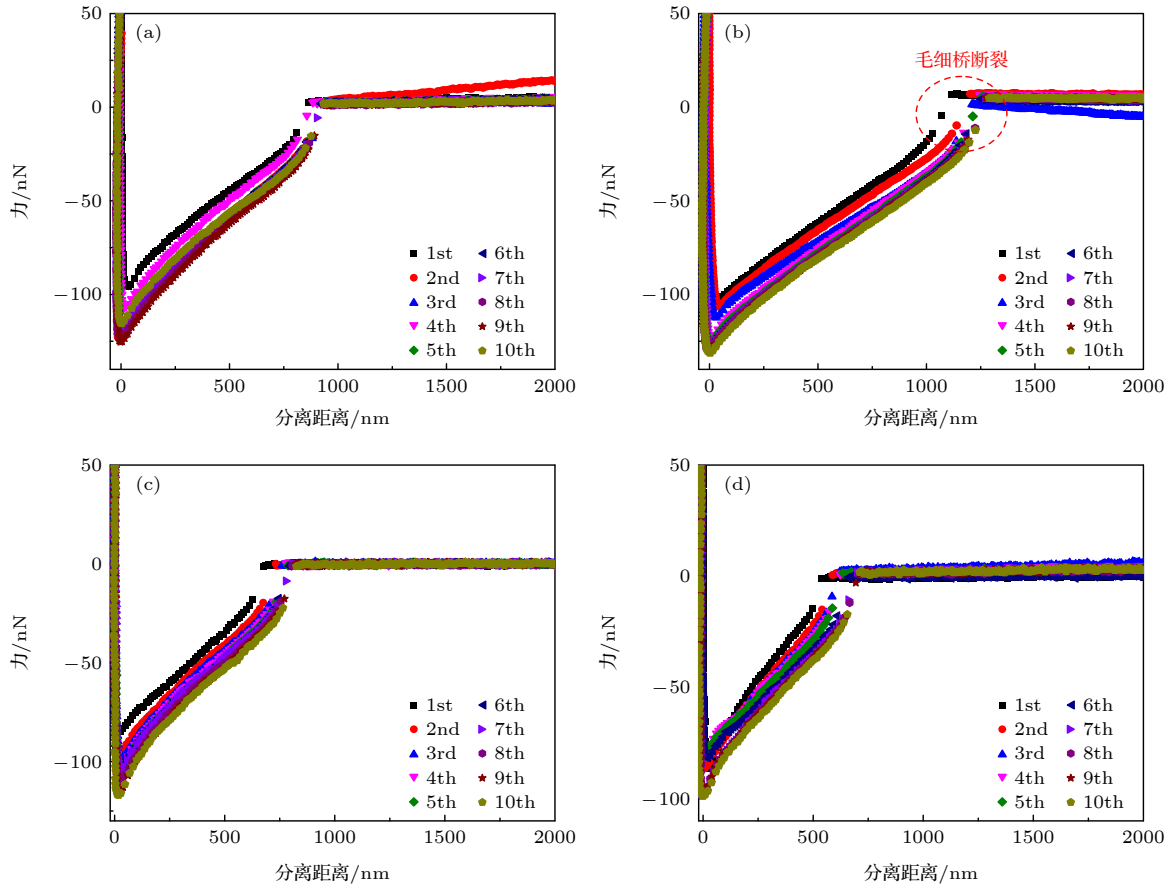
图 9 不同接近次数下的疏水颗粒与基板间相互作用力(退针曲线) (a) 位置 1; (b) 位置 2; (c) 位置 3; (d) 位置 4 Fig. 9. Interaction between hydrophobic particles and substrate under different approaching times (retraction curves): (a) Position 1; (b) position 2; (c) position 3; (d) position 4.
