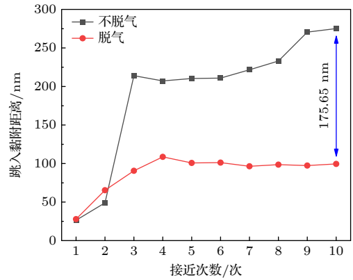
图 11 不同接近次数下进针跳入黏附距离变化 Fig. 11. Variation of adhesive distance upon penetration at different approaching cycles.
