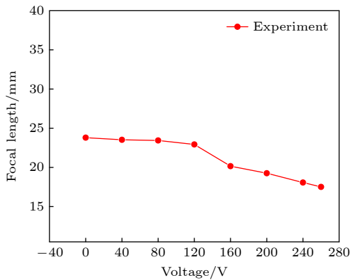
图10 不同电压下的双凸液体透镜焦距图
