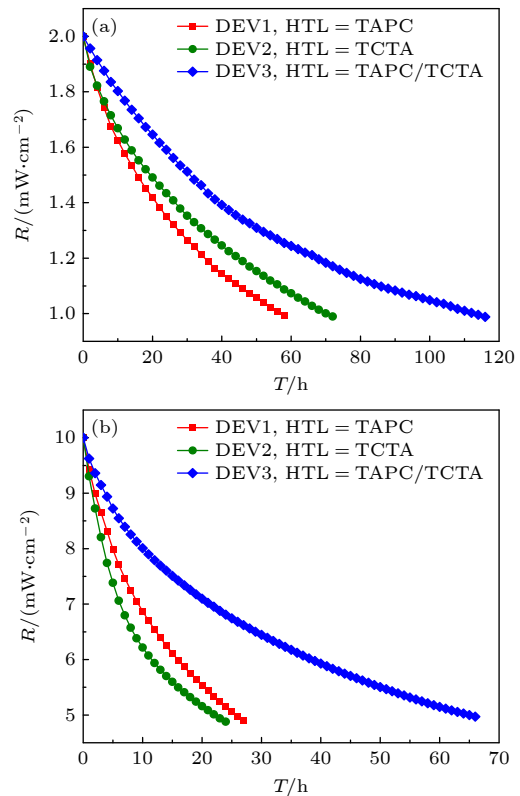
图 5 DEV1, DEV2, DEV3 在两种恒压模式下的稳定性对比 (a) R_0 = 2 mW/cm 2 ; (b) R_0 = 10 mW/cm 2
