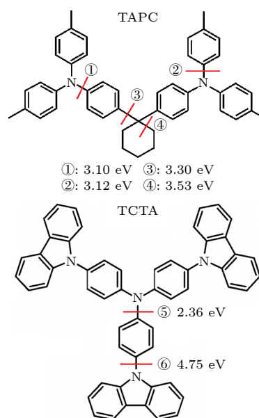
图 6 TAPC 与 TCTA 的分子结构与化学键解离能 Fig. 6. Molecular structures and bond dissociation energies of TAPC and TCTA molecules.
