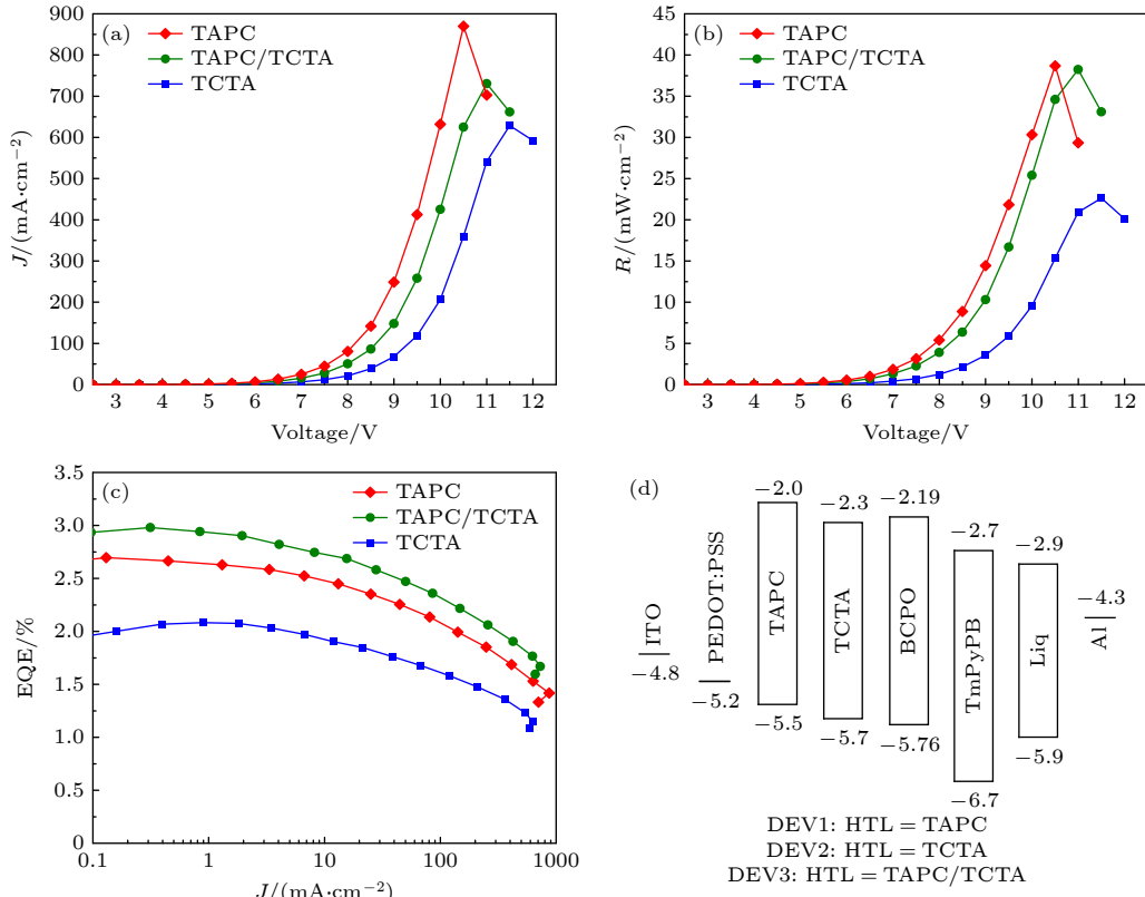
图 4 具有不同空穴传输层器件的性能对比 (a) J - V 曲线; (b) R - V 曲线; (c) EQE- J 曲线; (d) 器件结构图
