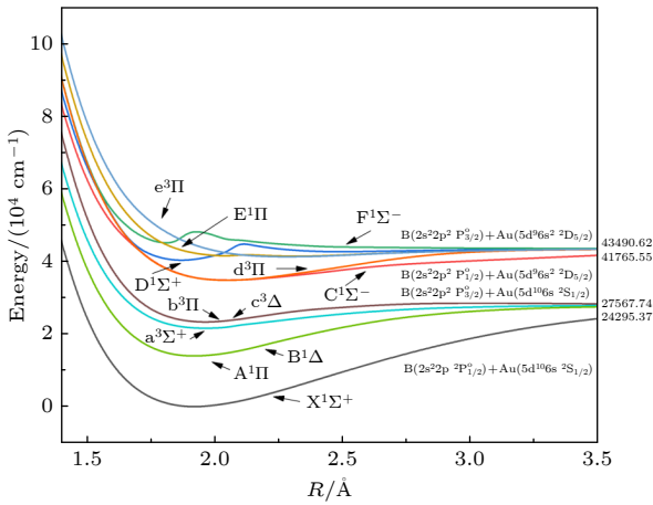
图 1 基于多参考组态相互作用方法计算的 AuB 分子 12 个 \Lambda -S 态的势能曲线随原子核间距的变化
