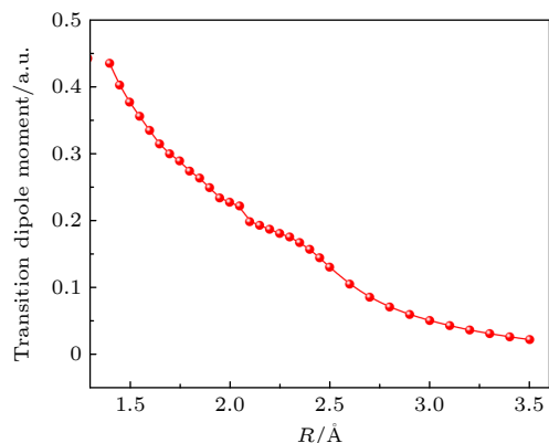
图 5 AuB 分子态跃迁 A^1\Pi_1 - X^1\Sigma_{0+} 的跃迁偶极矩随核间距的变化
