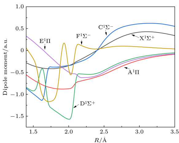
图 2 AuB 分子的 6 个单重态偶极矩随核间距的变化, 电子态分别为 \text{X}^1\Sigma^+ , \text{A}^1\Pi , \text{C}^1\Sigma^- , \text{F}^1\Sigma^- , \text{E}^1\Pi 和 \text{D}^1\Sigma^+
