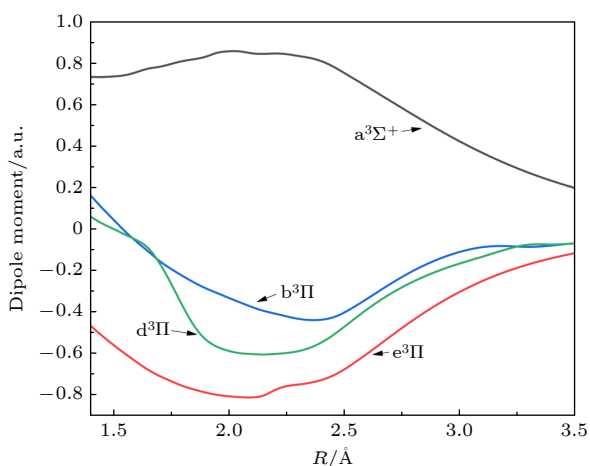
图 3 AuB 分子的 4 个三重态偶极矩随核间距的变化, 电子态分别为 \text{a}^3\Sigma^+ , \text{b}^3\Pi , \text{d}^3\Pi 和 \text{e}^3\Pi
