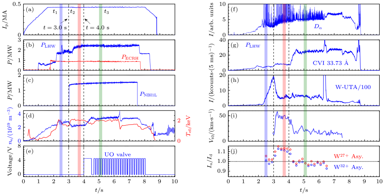
图 3 EAST #93801 放电波形图 (a) 等离子体电流 I_p ; (b) 低杂波加热功率 P_{\text{LHW}} 及电子回旋加热功率 P_{\text{ECRH}} ; (c) 中性束加热功率 P_{\text{NBILL}} ; (d) 弦平均电子密度 n_e 和芯部电子温度 T_{e0} ; (e) O 窗口上外充气口的充气阀门电压; (f) 上偏滤器 D_\alpha 信号; (g) CVI ( \text{C}^{5+} , 33.73 Å) 线辐射强度; (h) 钨未分解跃迁系辐射强度 (W-UTA, 45—70 Å); (i) 芯部环向旋转速度 V_{t0} ; (j) \text{W}^{27+} 51.457 Å, \text{W}^{32+} 52.2 Å 线辐射不对称性因子 I_u/I_d
