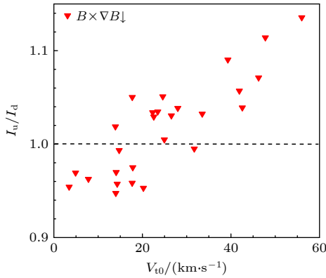
图 5 W^{32+} 52.2 Å 线辐射强度不对称因子 I_u/I_d 随芯部环向旋转速度 V_{t0} 的变化
