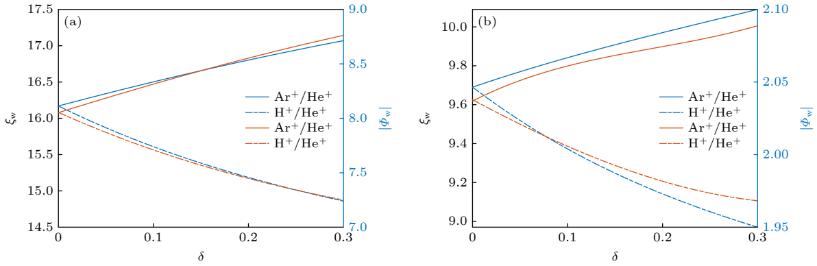
图 11 杂质离子种类、浓度和非广延参量对鞘层厚度和壁面电势的影响 ( B = 0.06 , \theta = 15^\circ ) (a) q = 0.7 ; (b) q = 1.3
