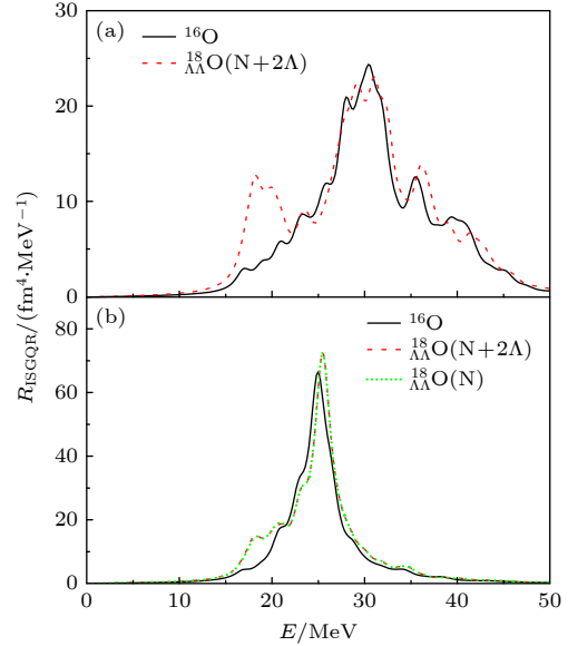
图 3 ^{16}\text{O} 和 ^{18}_{\Lambda\Lambda}\text{O} 的同位旋标量巨四极共振响应函数 (a) Hartree 响应函数; (b) RRPA 响应函数
