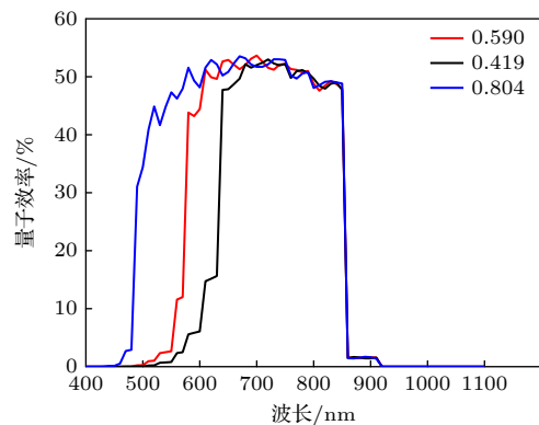
图 3 量子效率随 Al 组分的变化
