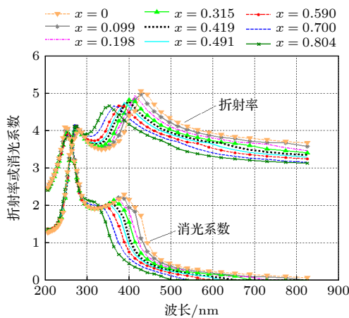
图 2 Ga_{1-x}Al_xAs 光学常数随 Al 组分的变化 [10]
