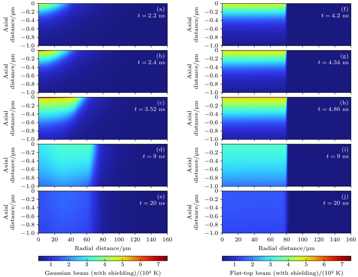
图 5 F = 20 \text{ J/cm}^2 , 考虑等离子体屏蔽时, 不同时刻的靶材温度分布 (a)–(e) 高斯光束烧蚀结果; (f)–(j) 平顶光束 ( r_1 = 1.2\omega_0 ) 烧蚀结果; 其中, (a), (f) 代表靶材蒸发开始时刻; (b), (g) 代表高温开始时刻; (c), (h) 代表高温结束时刻; (d), (i) 代表靶材蒸发结束时刻; (e), (j) 代表靶材仿真结束时刻
