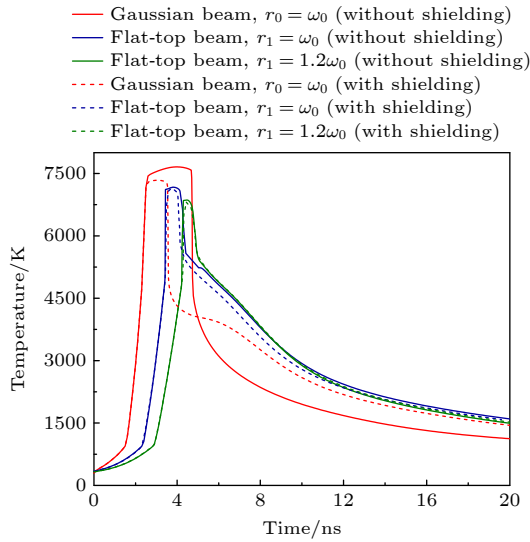
图 4 F = 20 \text{ J/cm}^2 , 靶面中心温度随时间的演化
